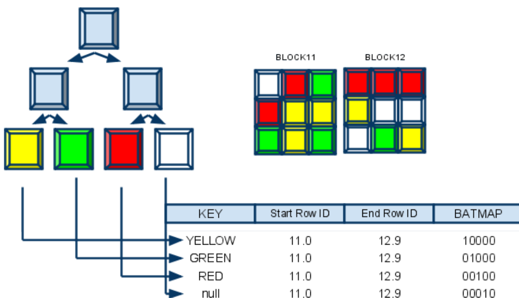
Рис. 3.4: Битовый индекс
