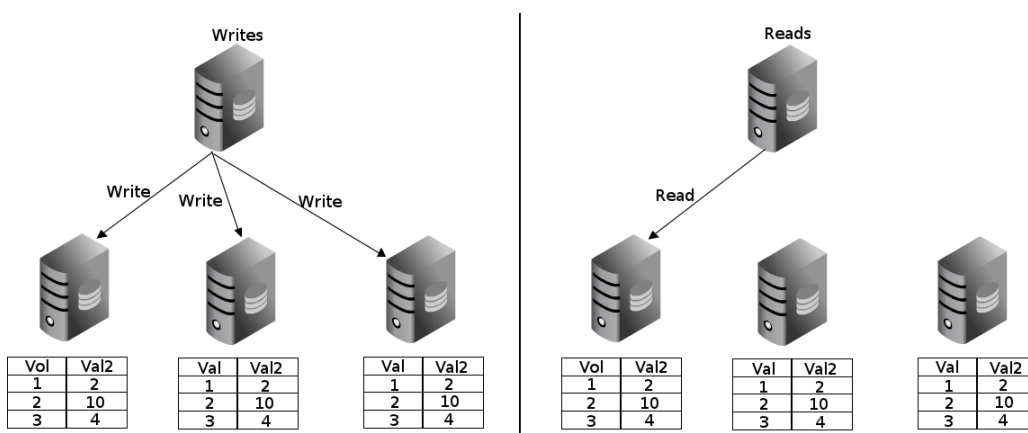
Рис. 6.3: Реплицированные таблицы
