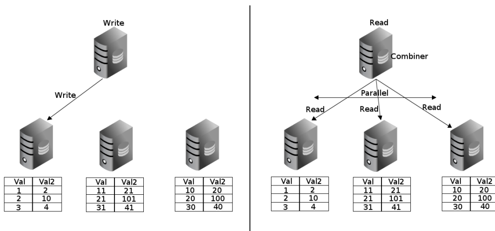
Рис. 6.2: Распределенные таблицы
